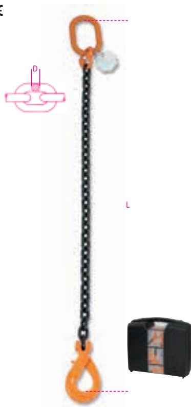
UNI EN 818-4
