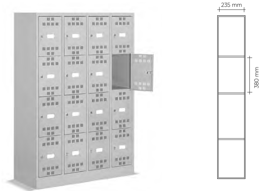
Esempio a 16 scomparti
