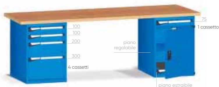
Armadio dim. mm 561x726x800 H (27x36 EH)
