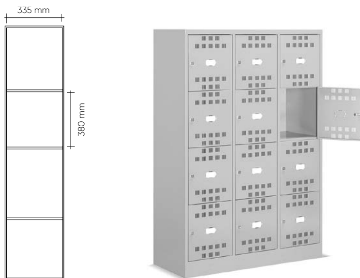
Esempio a 12 scomparti
