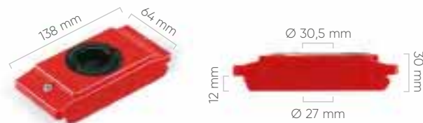
BOCCOLA HSK A40-B50
